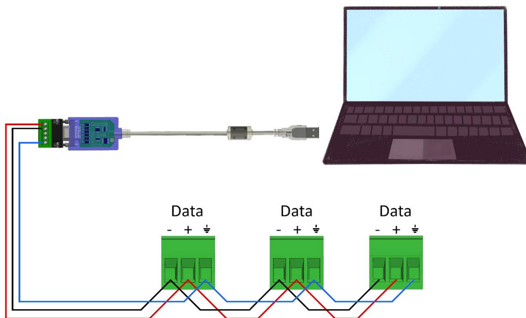
Figura 22 - Esquema de Ligação RS-485
