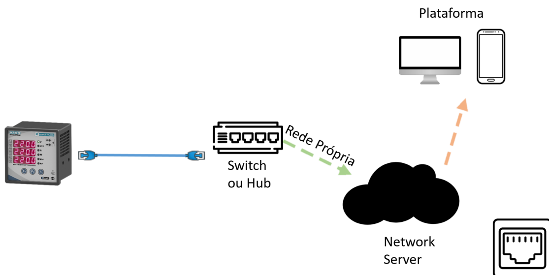
Figura 89 - Conexão Ethernet
