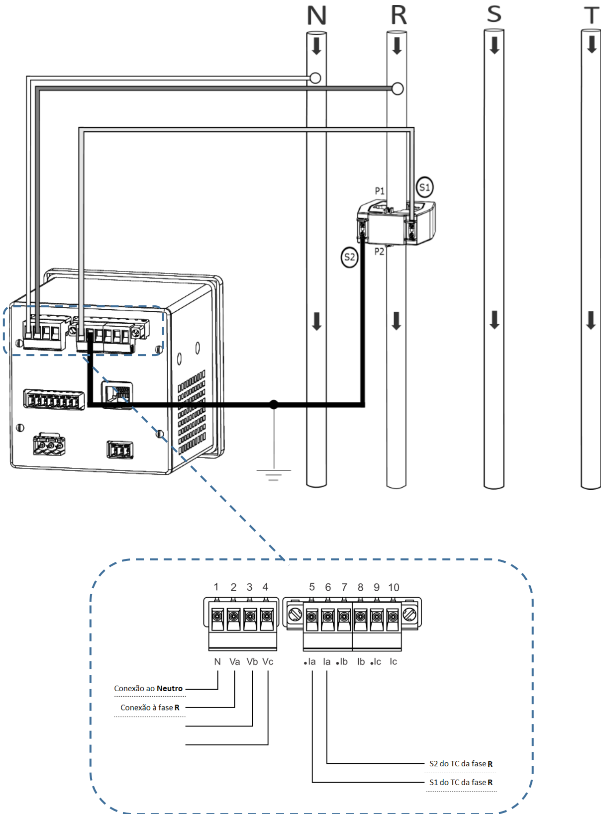
Figura 15 - TL03 Trifásico Equilibrado
