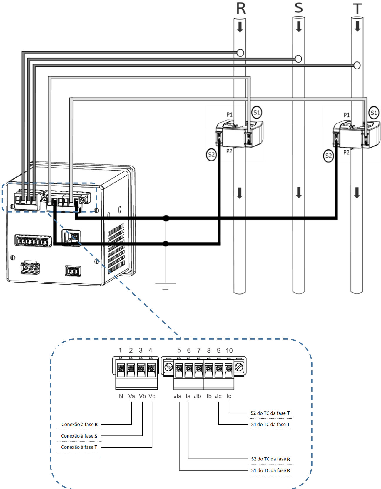
Figura 14 - TL17 Trifásico Equilibrado Delta
