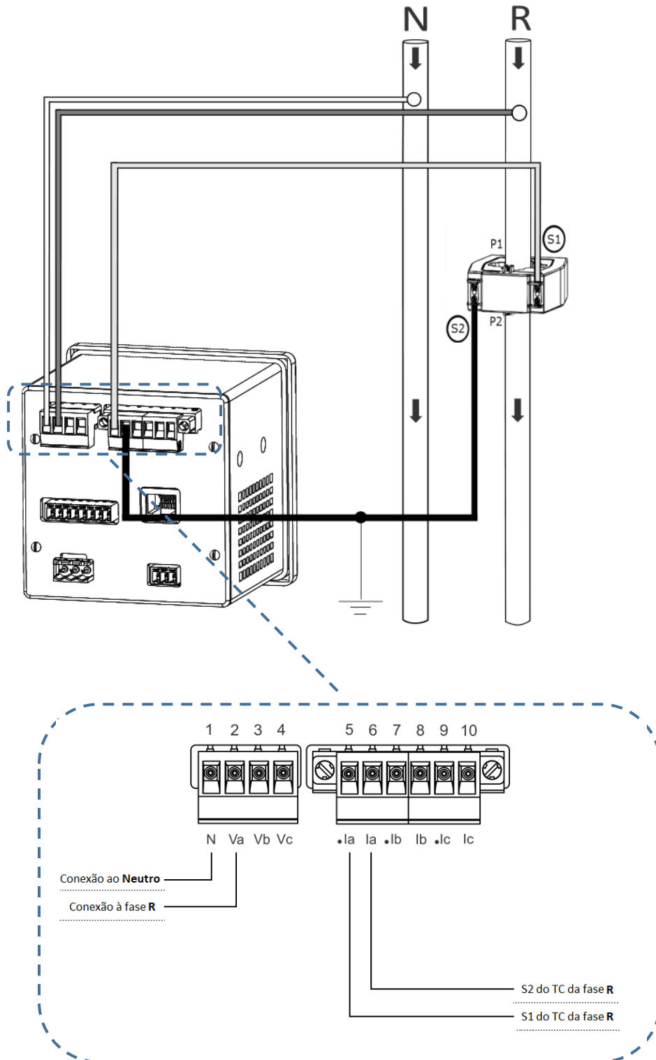
Figura 10 - TL02 Monofásico
