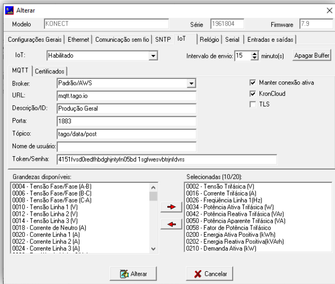
Figura 74 - IOT
