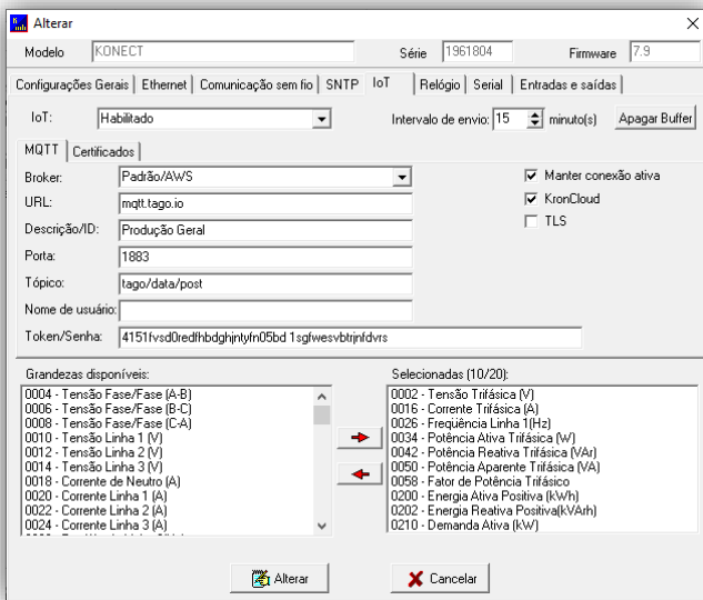
Figura 49 - IOT
