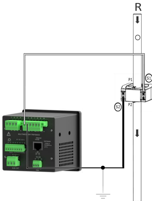
Figura 9 - Entrada de Corrente
