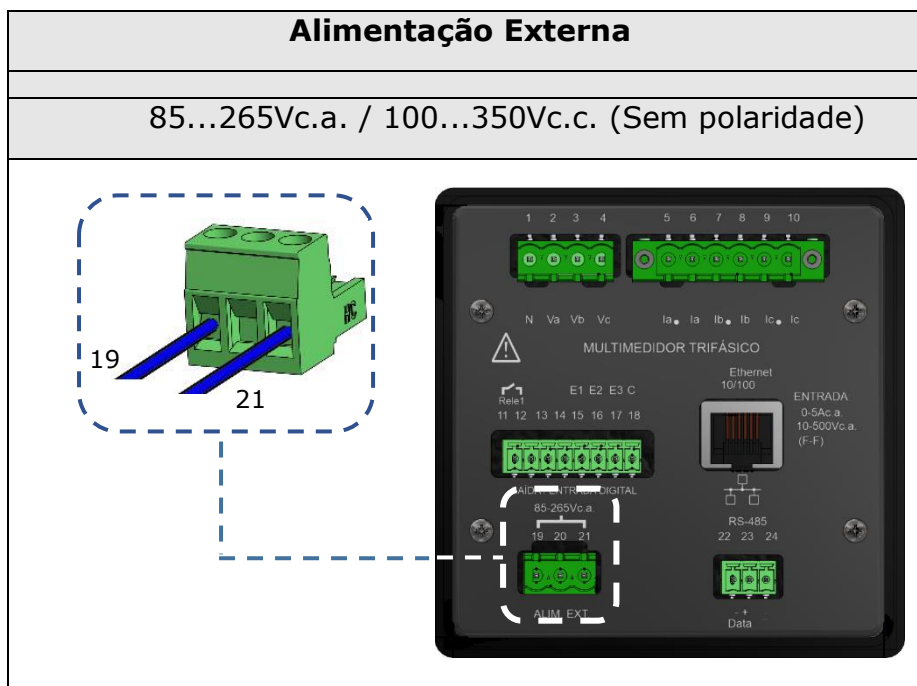
Figura 6 - Alimentação Externa
