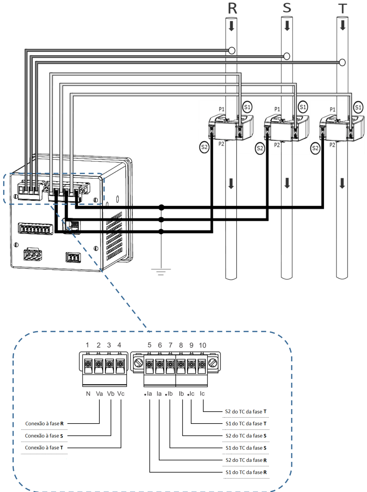
Figura 13 - TL48 Trifásico Delta
