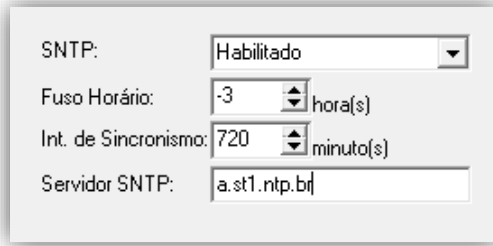
Figura 48 - SNTP
