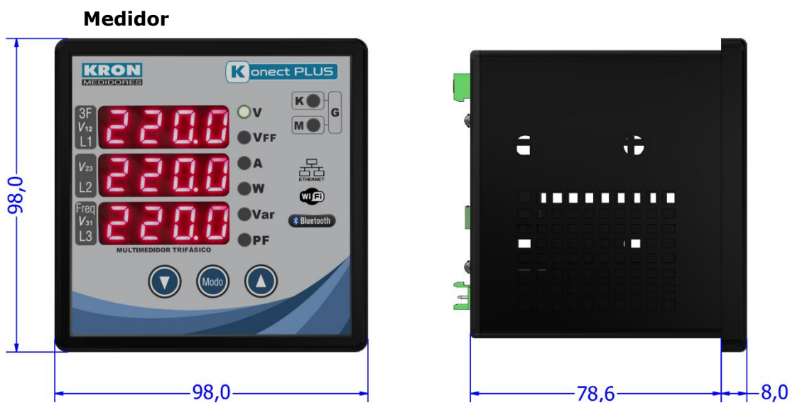
Figura 2 - Dimensionais
