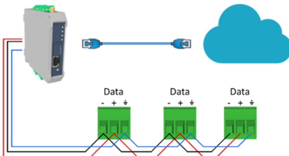
Figura 24 - Esquema de Ligação Gateway K-GTWB
