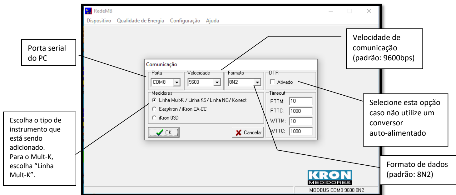
Configuração da porta serial
